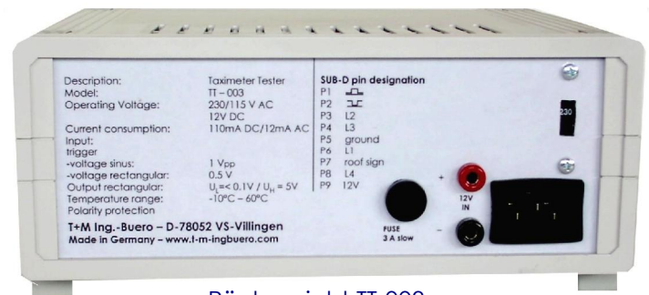
Rückansicht TT-003
